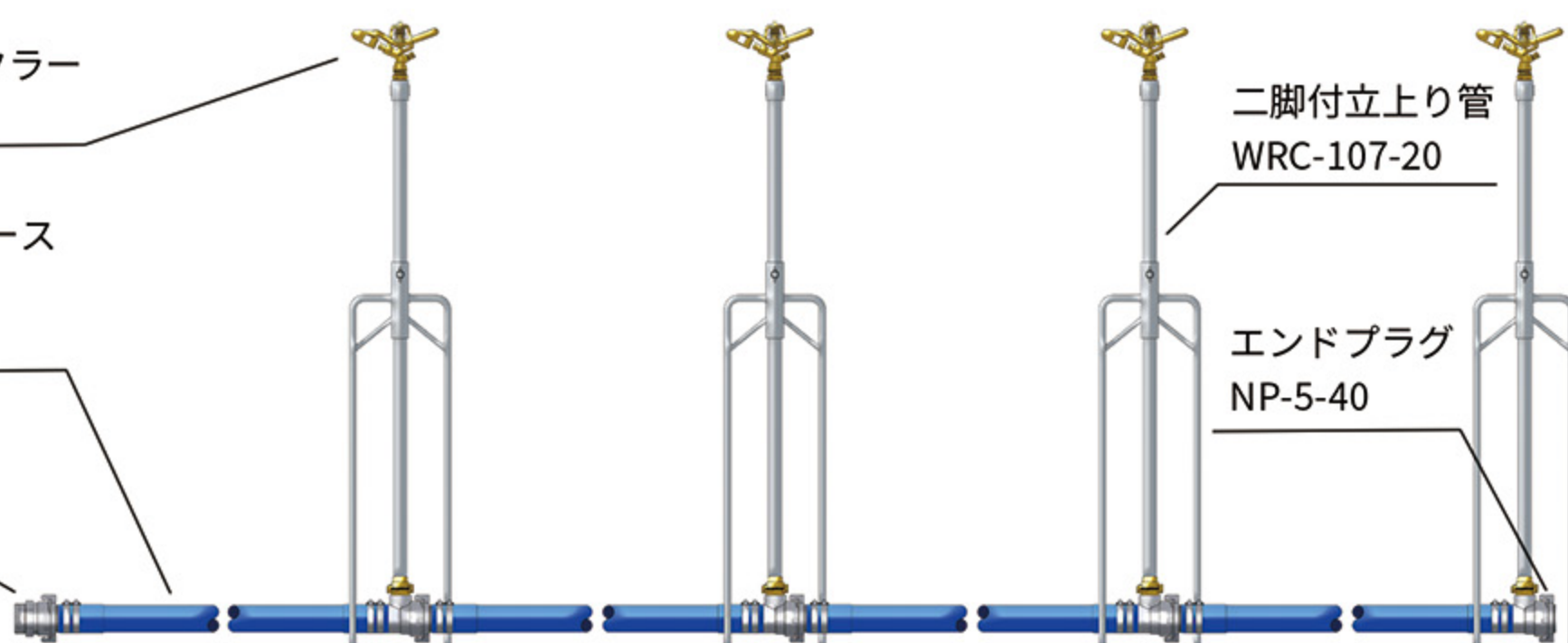
※NPC-404S6-W107 (40mm) 参考図
