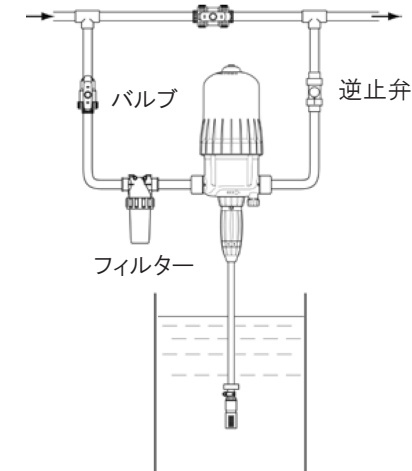
バイパス設置例
