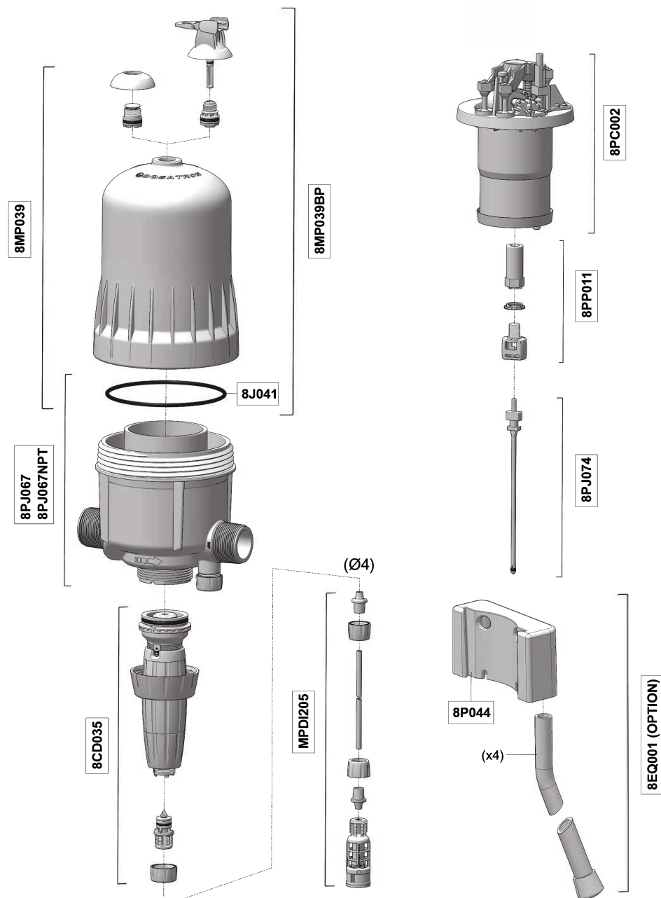
主パーツ図
