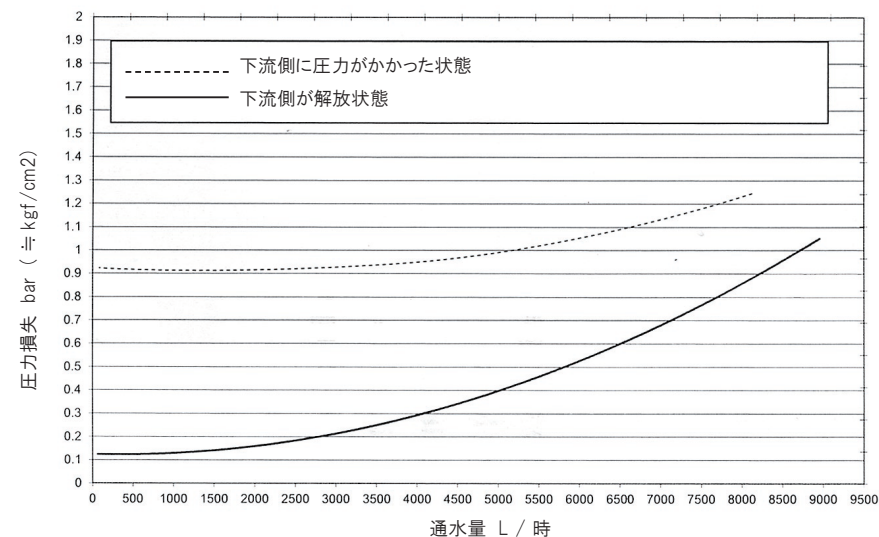
通水量による圧力損失表
