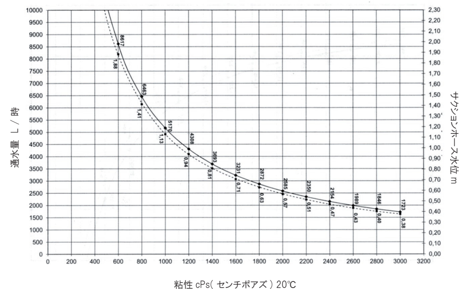
吸入液粘性によるサクシオン水位
