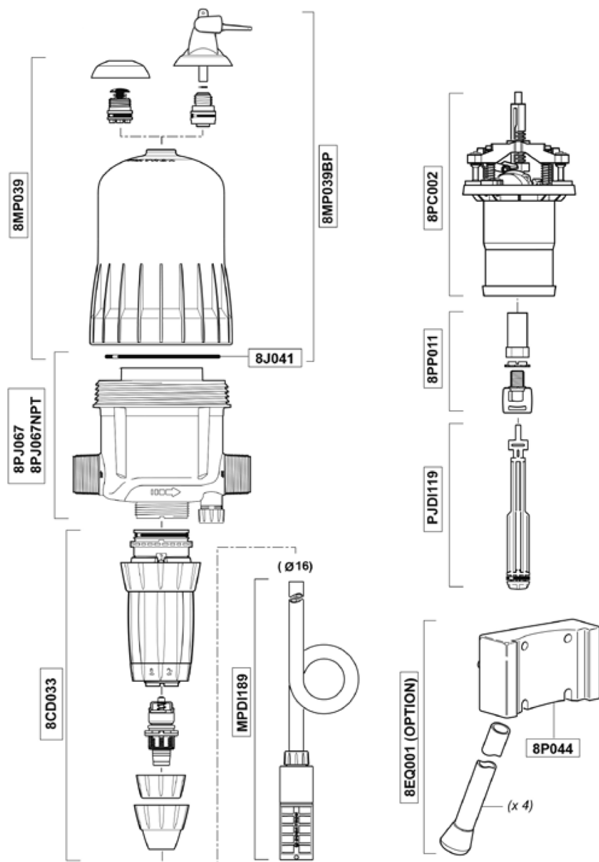
主パーツ図
